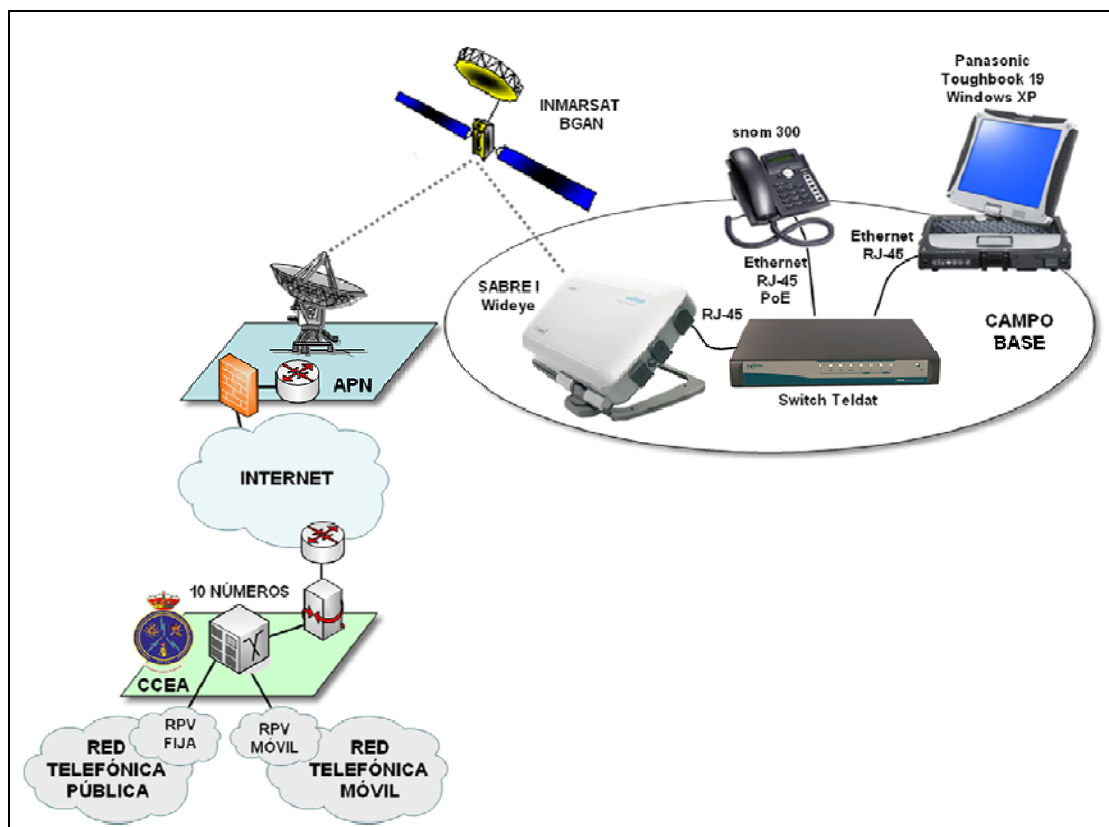
Figura 2. Integración en la RPV del Ministerio.
